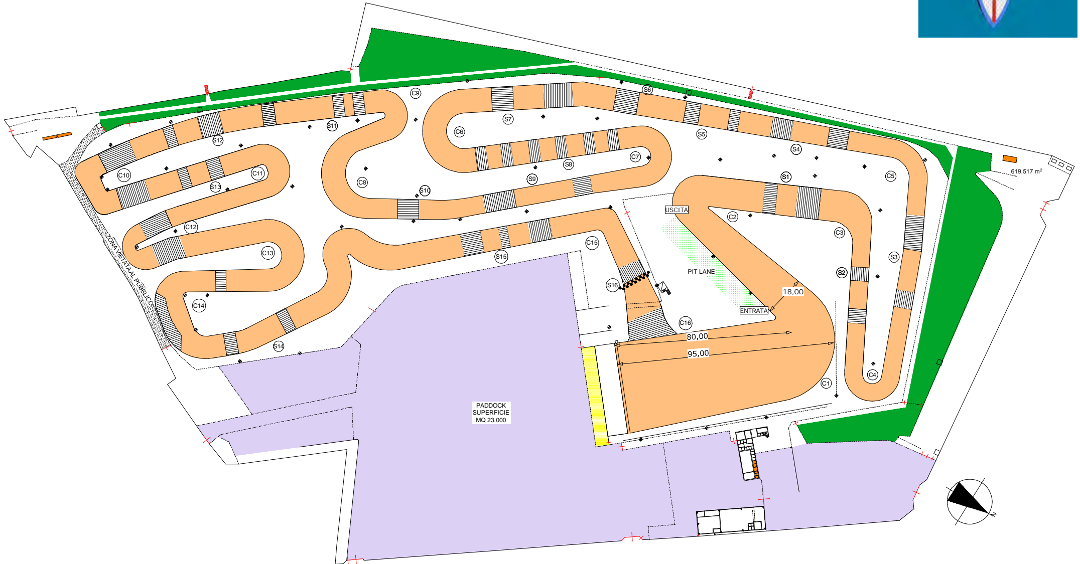
PLANIMETRIA NUOVA SOLUZIONE scala 1:1200
